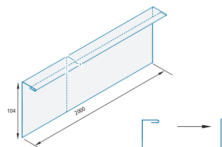
Bande à rabattre épaisseur : 0,65 mm ou 0,70 mm longueur : 2 m
