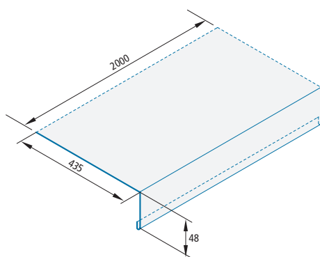
Bande d'entourage de baie épaisseur : 0,70 mm - longueur : 2 m
